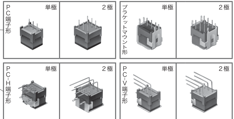
端子部形状
