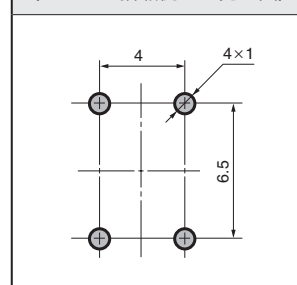
プリント基板取付寸法図 (スイッチ搭載側から見た図)
